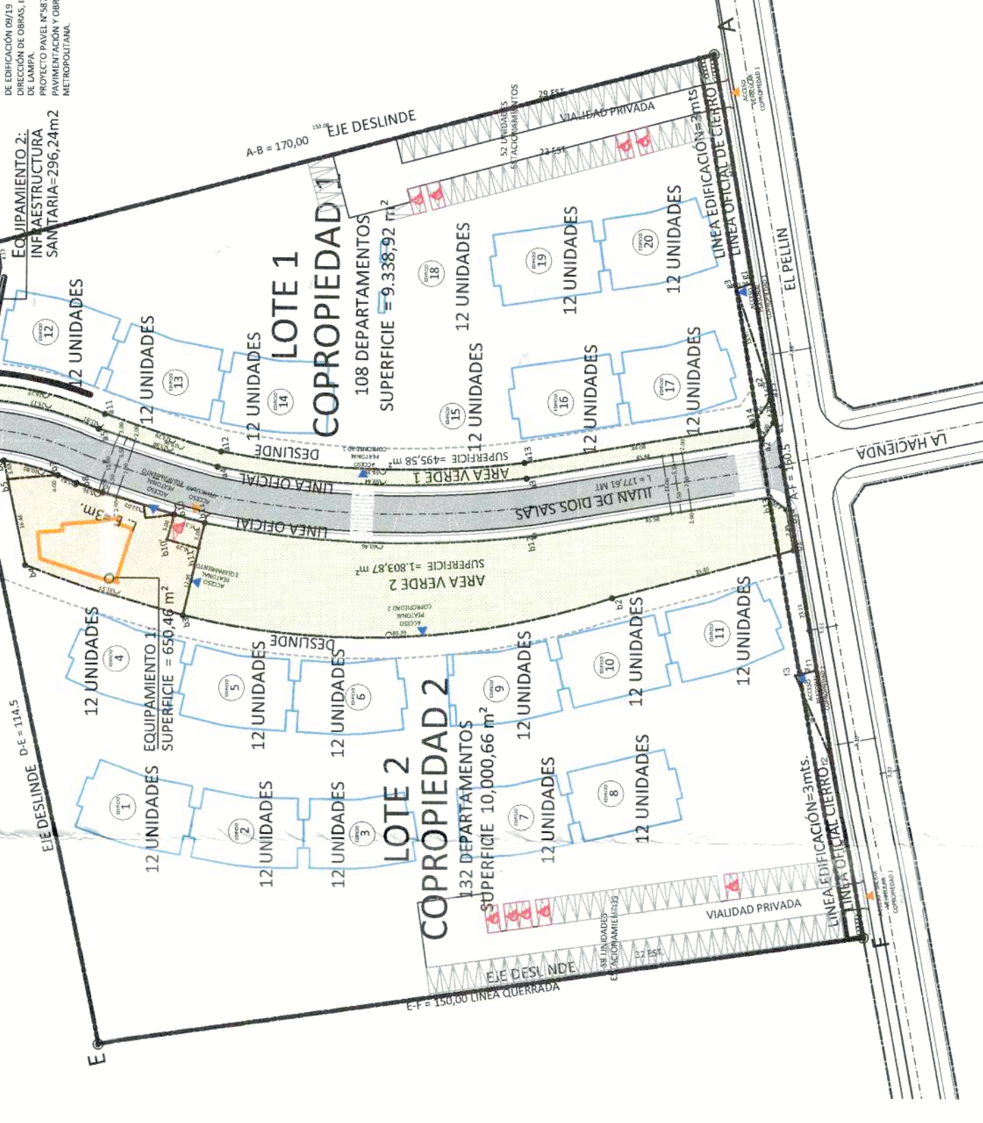
PLANTA DE EMPLAZAMIENTO LOTEJO: DENSIDADES ESC. 1 / 1.000
