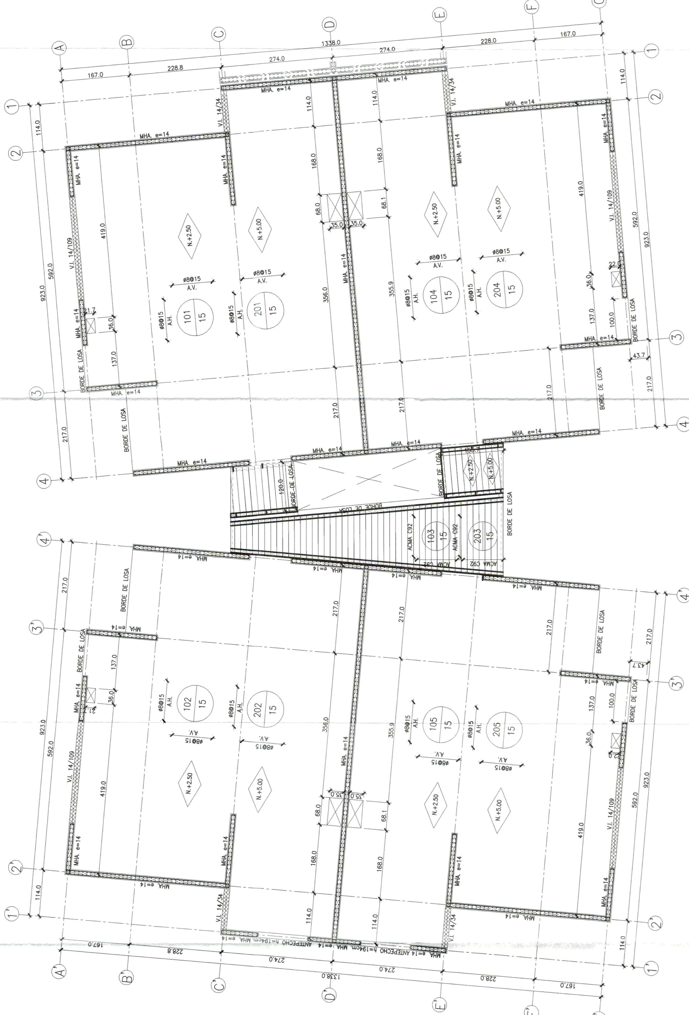
PLANTA DE ESTRUCTURA LOSA CIELO 1er Y 2do PISO. ESC: 1:50
