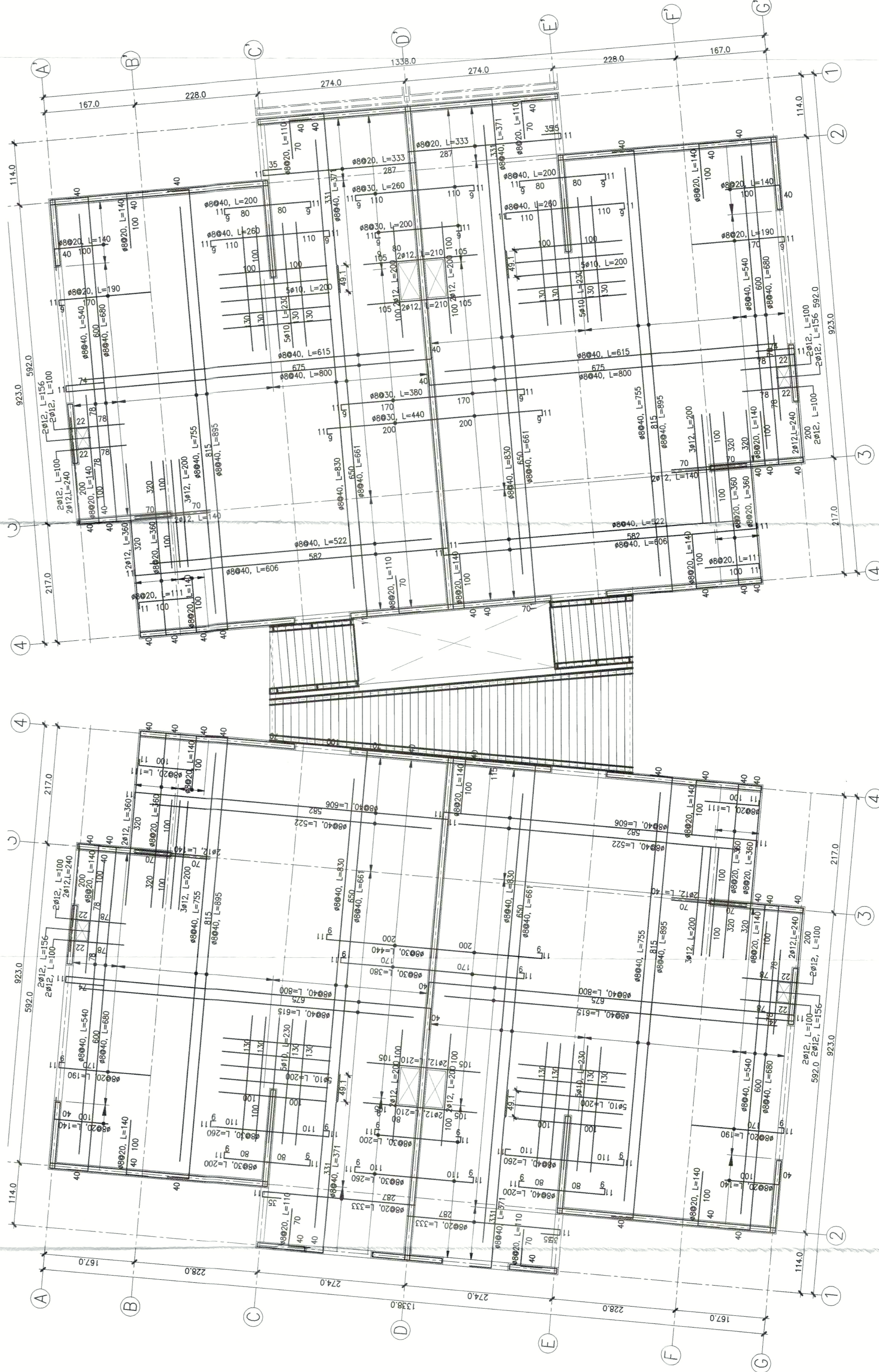
PLANTA DE ARMADURA LOSA CIELO 1er Y 2do PISO. ESC: 1:50
