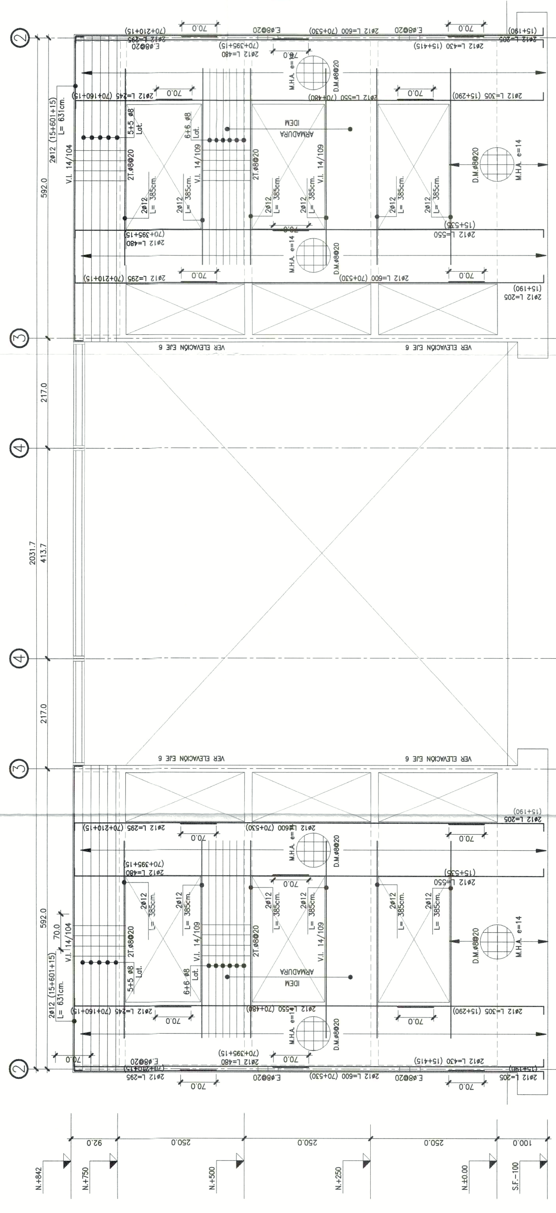
ELEVACION EJE G ESC. 1:50
