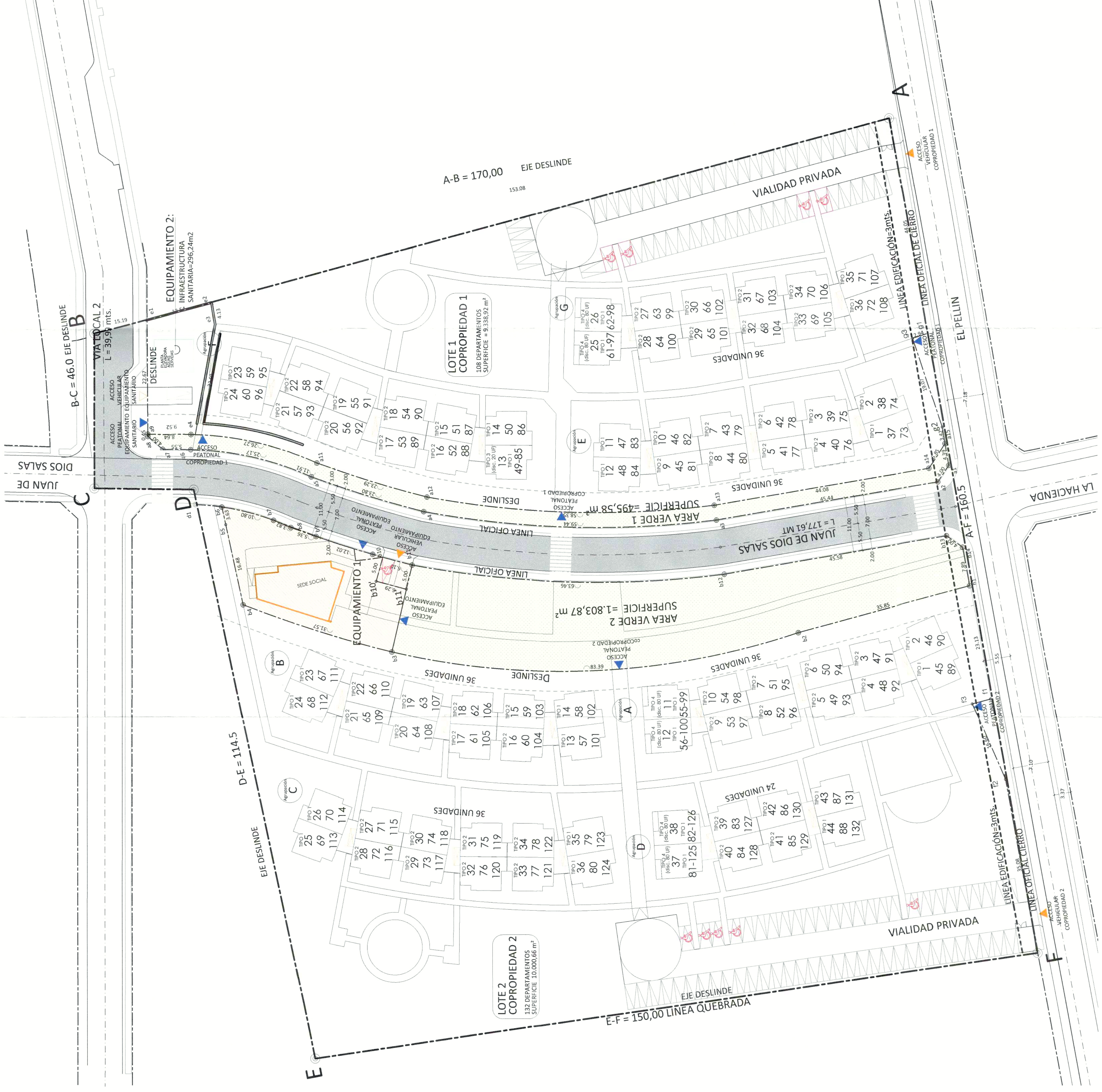
CONFIGURACION DE BLOQUES 1er AL 3er PISO: 240 DEPARTAMENTOS ESCALA 1/400
