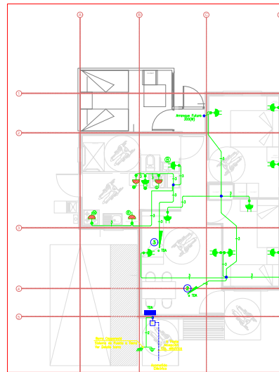
ENCHUFES VIVIENDA TIPO 4 1°PISO ESCALA: 1:50
