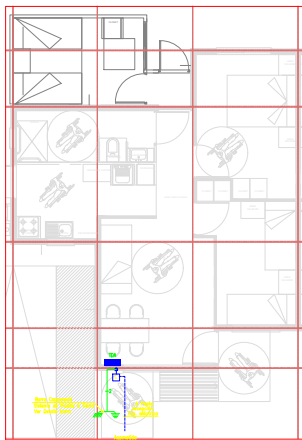
PUESTA A TIERRA VIVIENDA TIPO 3 1°PISO ESCALA: 1:50
