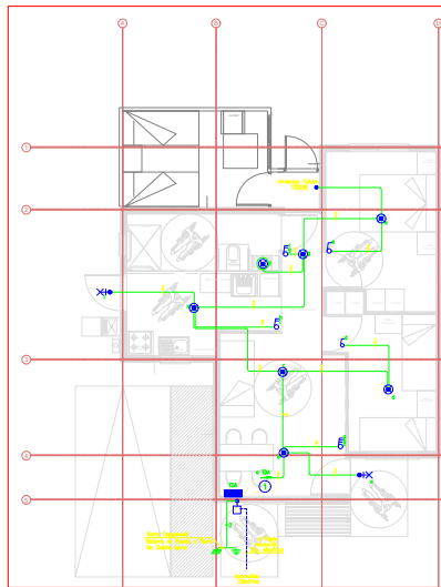
ALUMBRADO VIVIENDA TIPO 4 1°PISO ESCALA: 1:50
