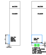
DETALLE TÍPICO CLOSET DEPTO. ESCALA: 1/25"
