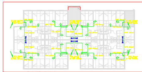
4° PISO (DUPLIX) EDIFICIO TIPO 2-3-4 ESCALA: 1/100"
