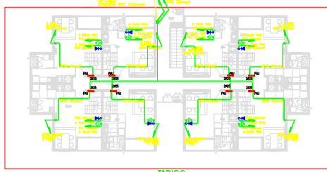
3° PISO EDIFICIO TIPO 1 ESCALA: 5/8"
