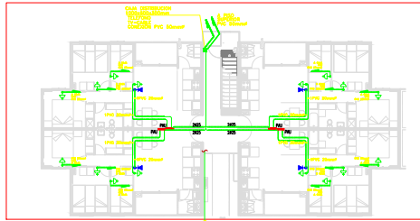
1° PISO EDIFICIO TIPO 1 ESCALA: 5/8"
