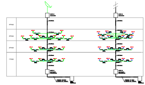
VERTICAL CORRIENTES DÉBILES DEPARTAMENTOS TIPO 1 ESCALA: 5/8"
