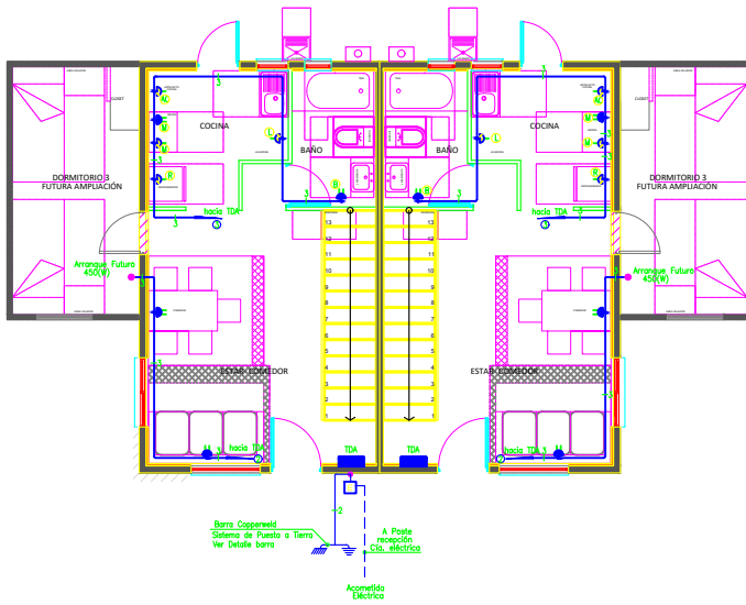
PLANTA 1° PISO MINUSVALIDOS SENSORIA ENCHUFES
