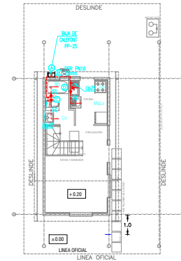
PLANTA VIVIENDA TIPO 7 1º PISO AGUA CALIENTE ESCALA = 1:100
