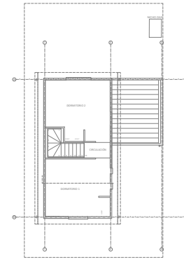
PLANTA VIVIENDA TIPO 7 2º PISO AGUA CALIENTE ESCALA = 1:100
