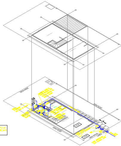
ISOMETRICO VIVIENDA TIPO 7 AGUA FRÍA ESCALA = 1:100
