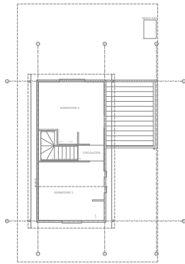
PLANTA VIVIENDA TIPO 7 2º PISO AGUA FRÍA ESCALA = 1:100
