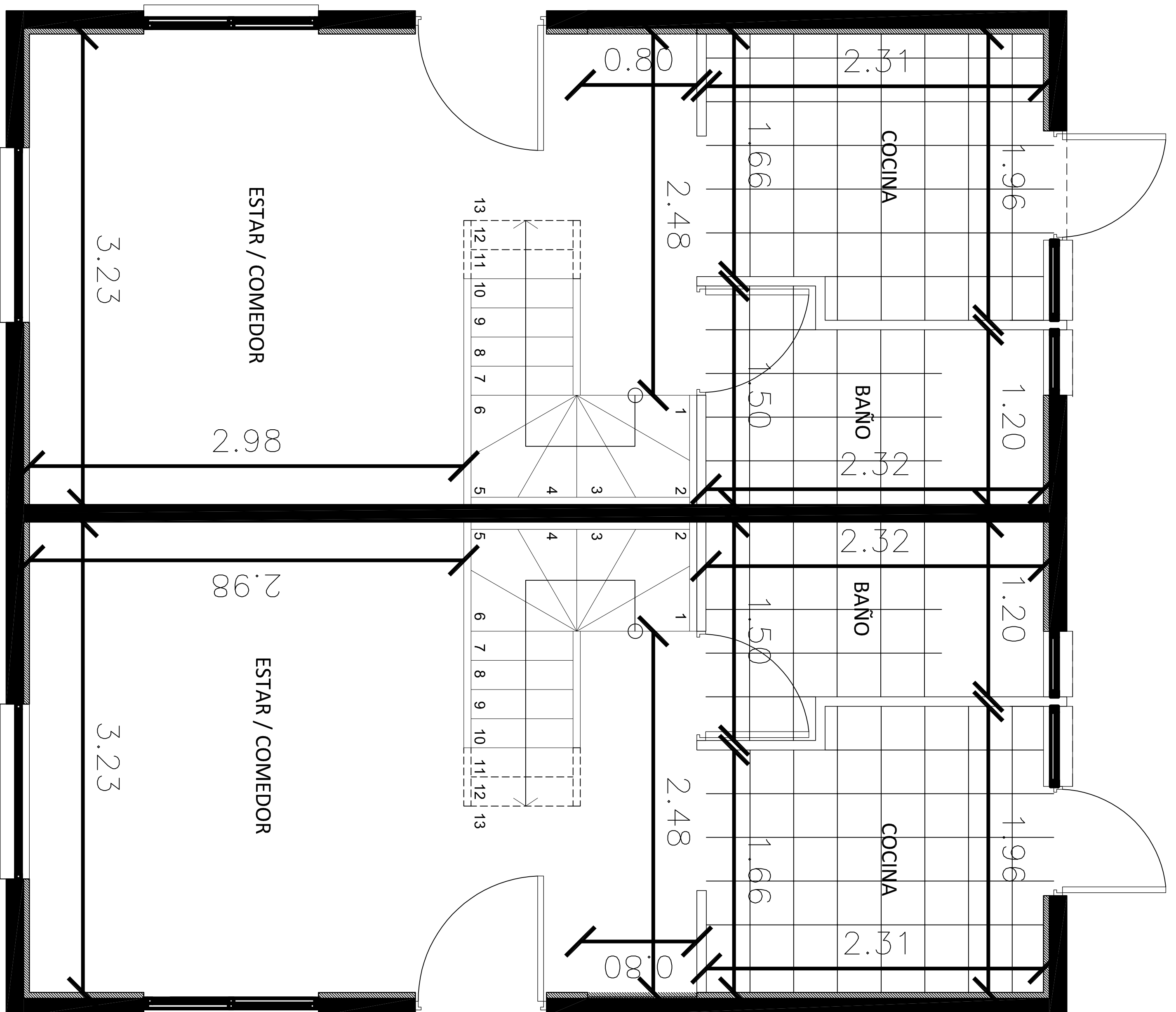
PISO 1
