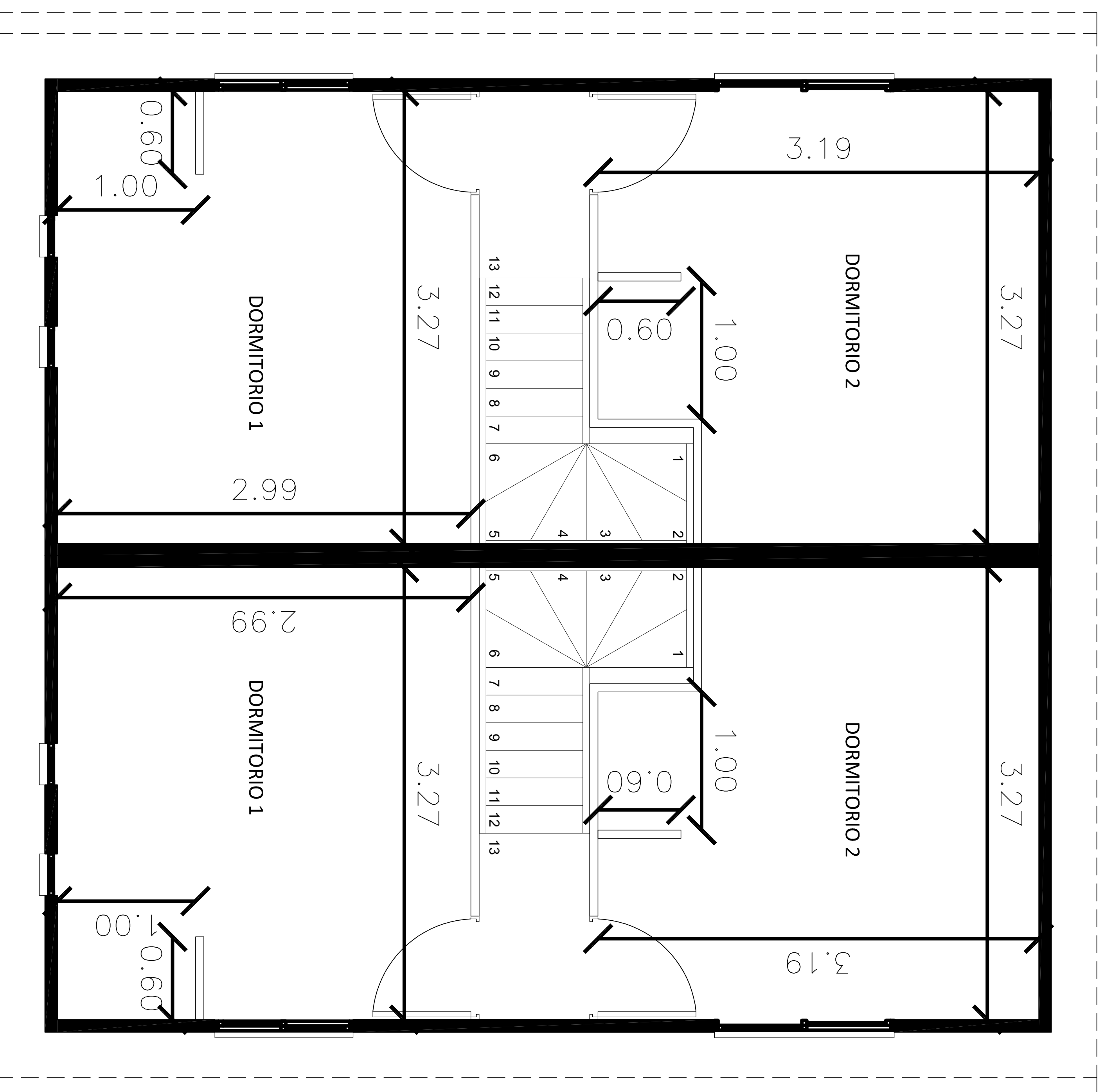
PISO 2
